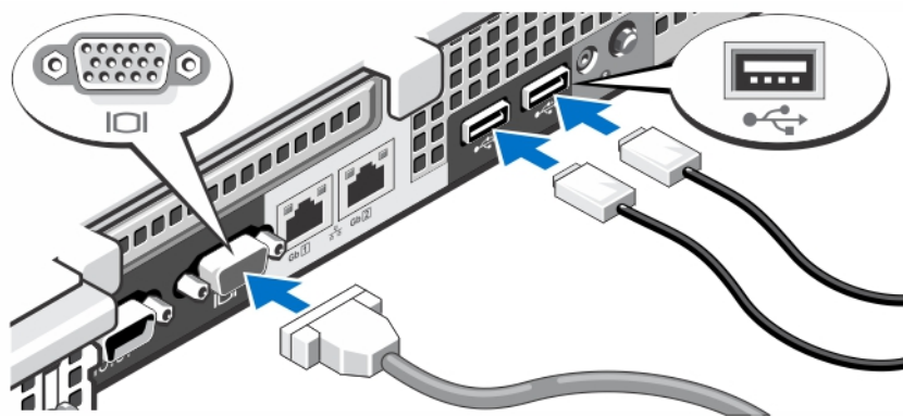
図2. オプション—キーボード、マウス、モニターの接続
